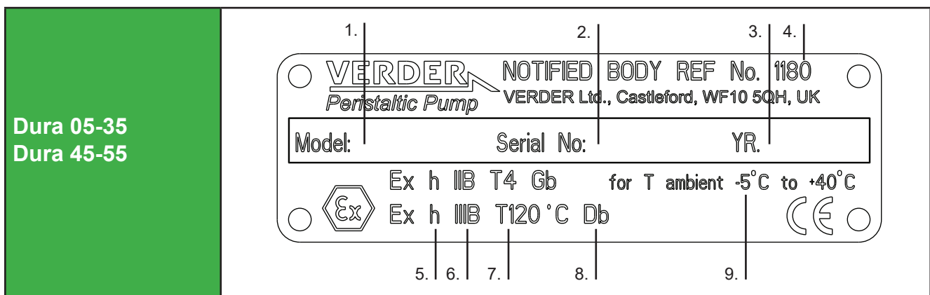
Figura 1 Placa Identificativa ATEX
